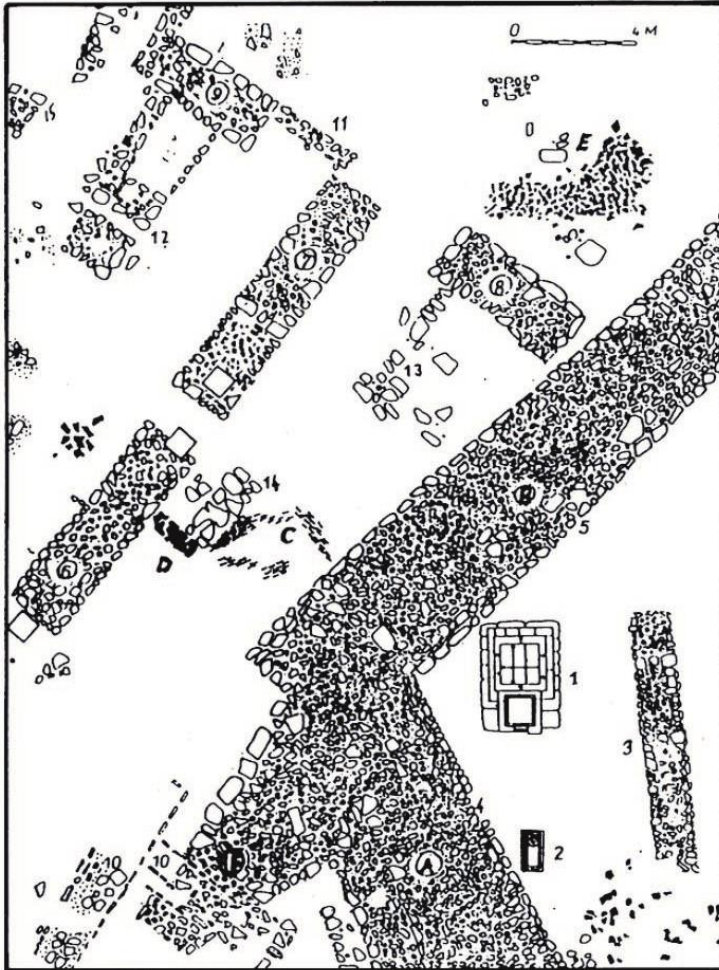
Fig. 3. DURAZZO. Planimetria dell'area di scavo.
