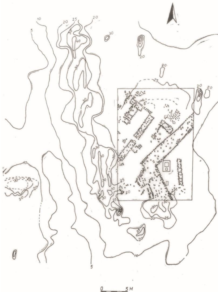
Fig 3. Harta e izovijave të rezistencës elektrike specifike
