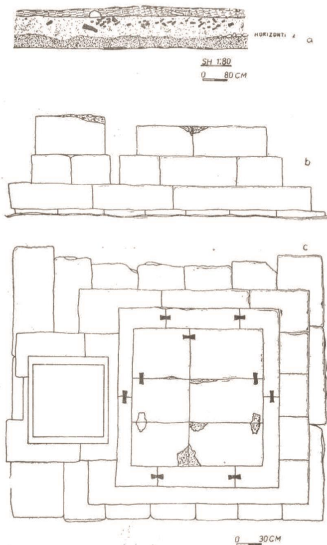
Fig 4. a – stratigrafia e altarit; b – prerje vertikale; c - planimetria
