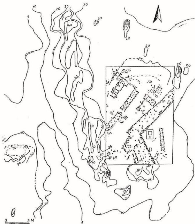
Fig 4. DURAZZO. Planimetria dell'area di scavo con le linee di resistenza elettrica specifica.
